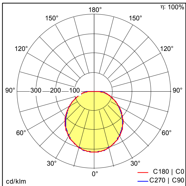
TE_LENA_VARIO_LED_380_2500_840.ltd
